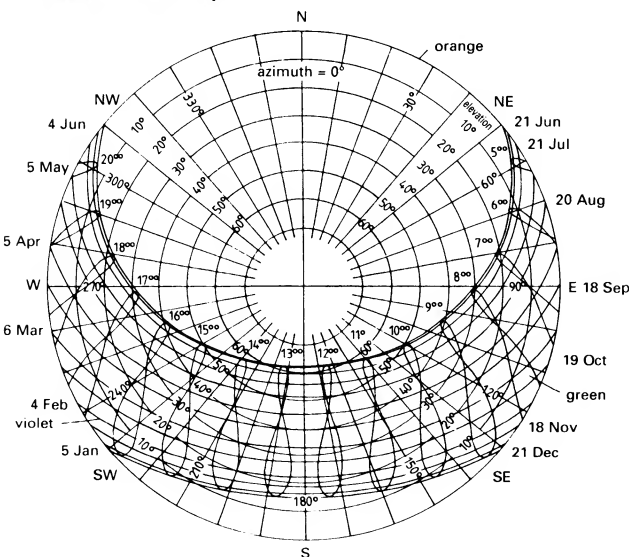
8 Solar position chart for latitude 49°52' N, longitude 8°39' W, time reference meridian: longitude 15°00' W
